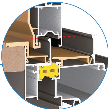
段差をなくし一段上の 水密性能を実現した 新下枠構造
