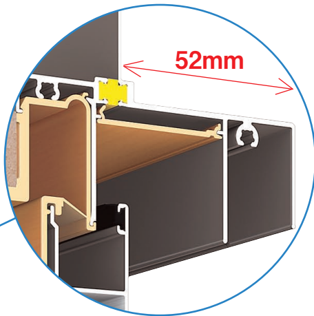
通気工法・厚壁化などに 対応できる 52mmのワイドな枠出幅
