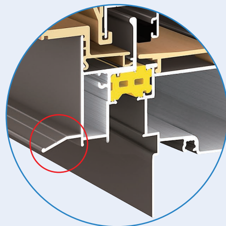
自重による前垂れを防ぐ 下枠固定フィン ※テラスタイプ
